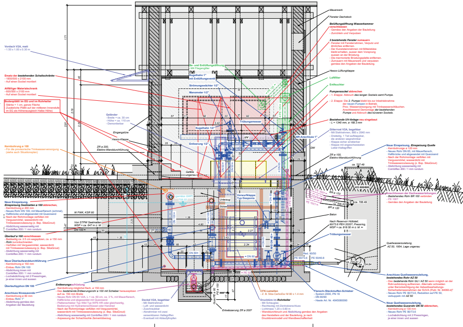
Schnitt A - A, 1 : 20
